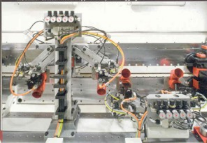
NOVIMAT Contour: neues Kapp- und Kopierfräsaggregat
